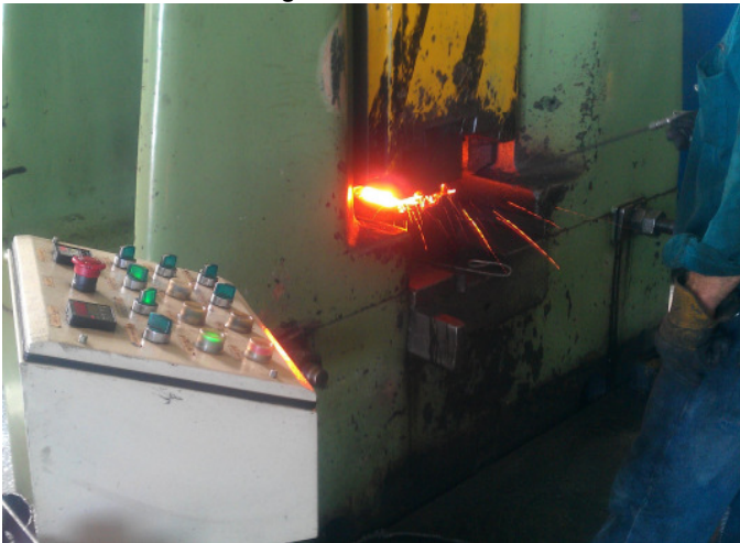
Warmpressen/Schmieden
