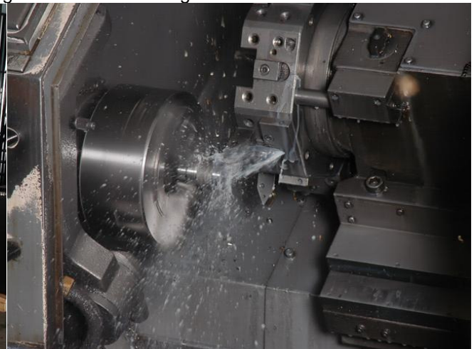
CNC Bearbeitung der Rohlinge
